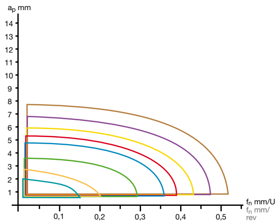
Längsdrehen 2,25D Longitudinal turning 2,25D
