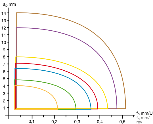
Längsdrehen 1,50D Longitudinal turning 1,50D
